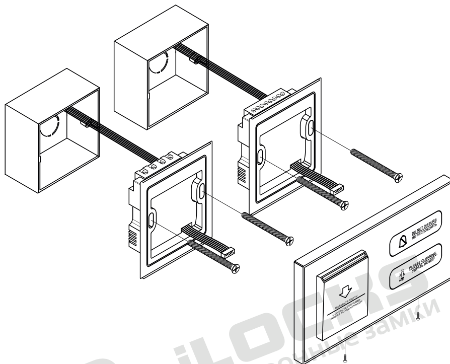
Рисунок №1 – Структурная схема (спецификация)
