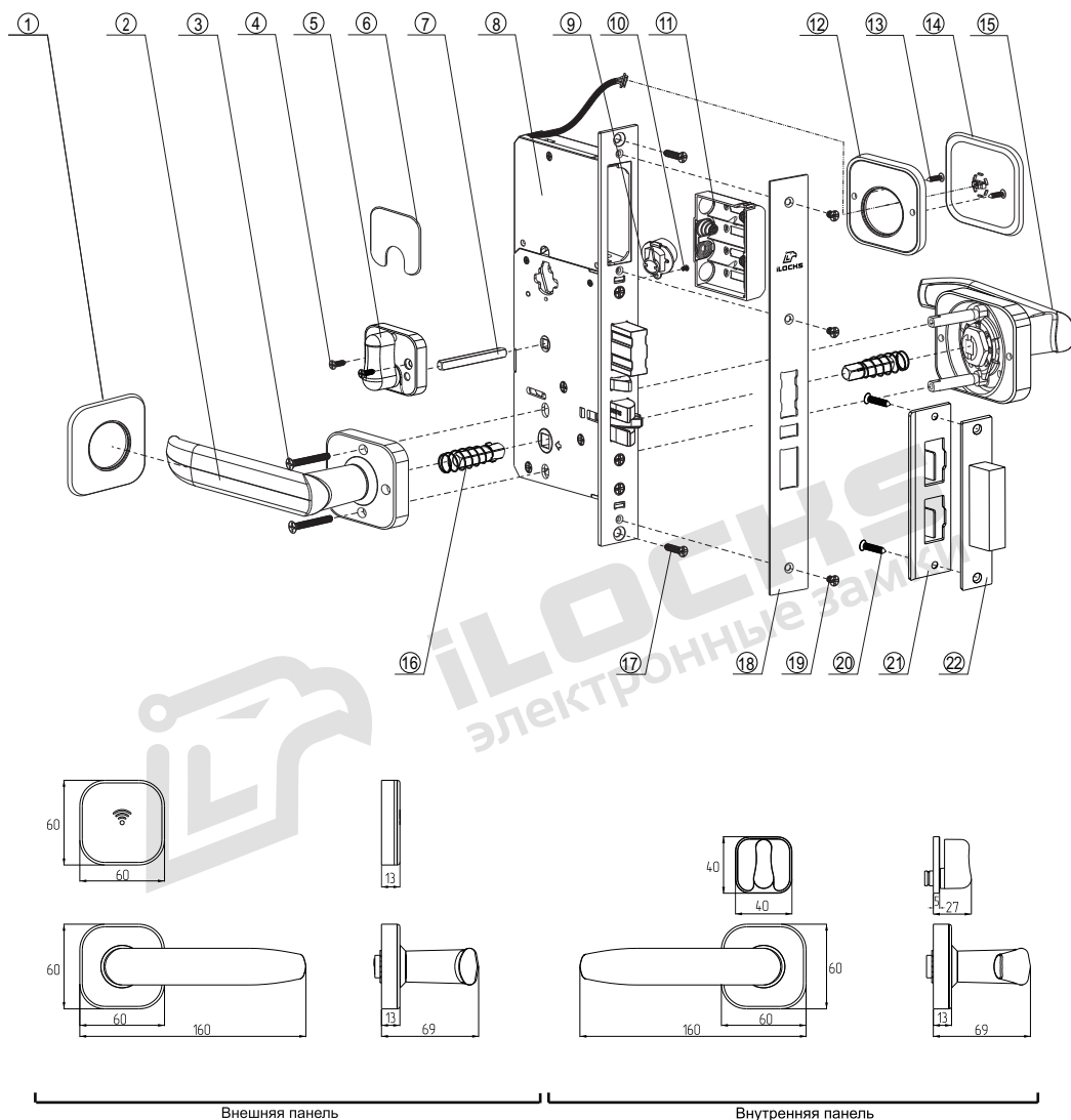
Рисунок №1 – Структурная схема (спецификация) замков типа iLOCKS IS170 433+BLE
