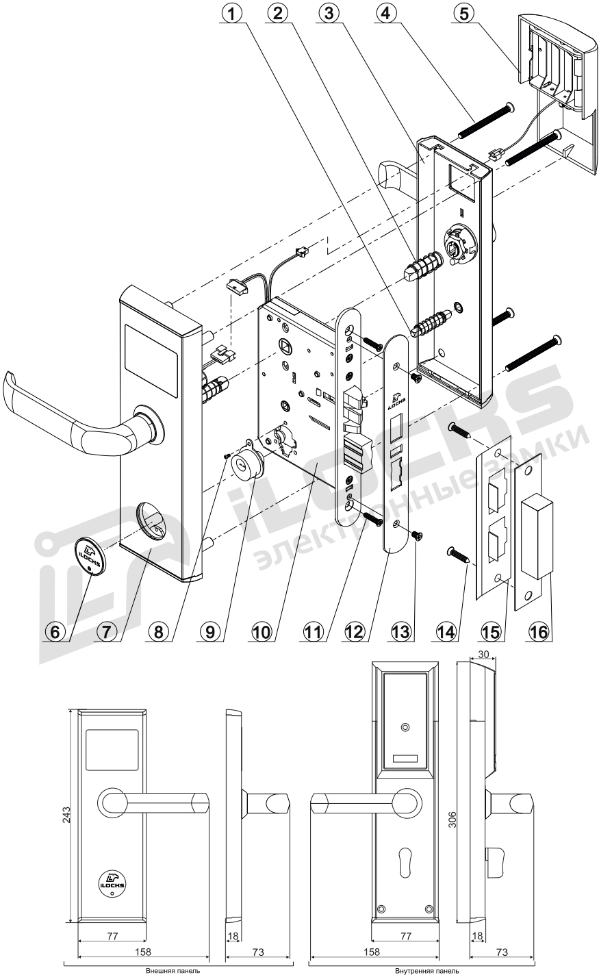
Рисунок №1 – Структурная схема (спецификация) замков и габариты замков типа iLOCKS IS8005A3B3
