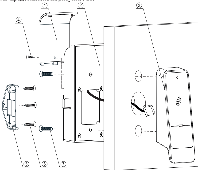
Рисунок №2 – Структурная схема (спецификация) замка IS0860-MF
